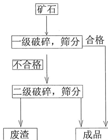
图 破碎工艺流程图
