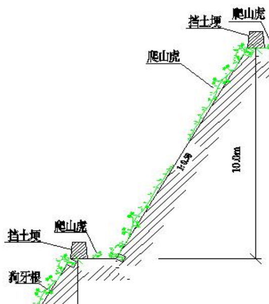
图 5-1 挡土墙示意图
