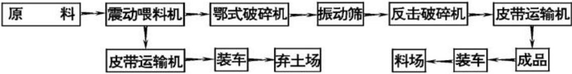
图 3-2 破碎工艺流程图
