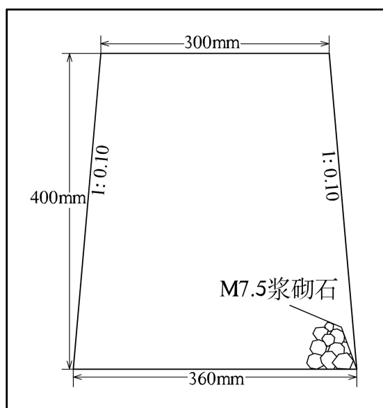
图 5-2 挡土墙断面设计示意图
