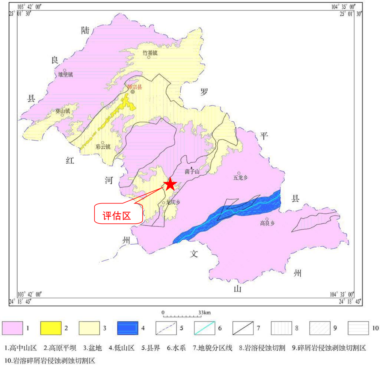
图 2-2 区域地貌图
