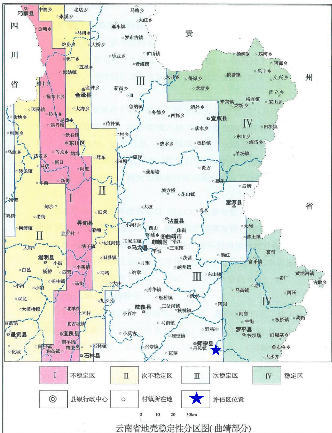
图 2-6 云南省地壳稳定性分区图
