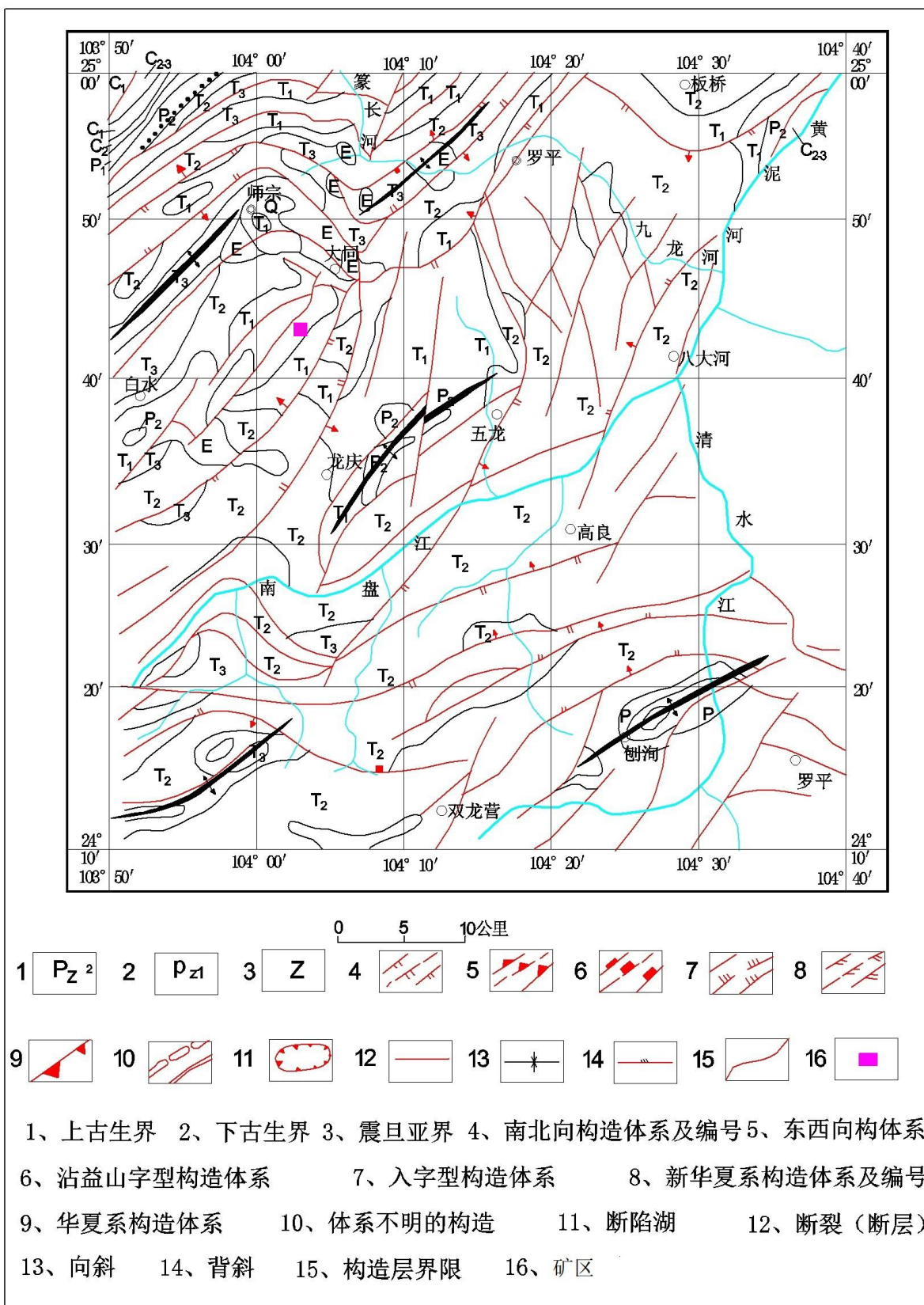
图 2-4 区域构造纲要图
