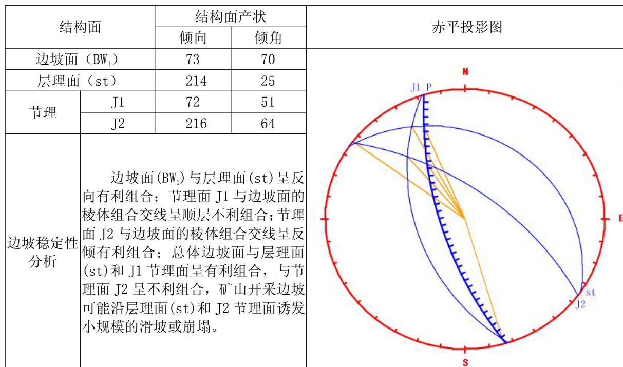
图 3-1 采场北部不稳定斜坡 (BW 1 ) 赤平投影图
