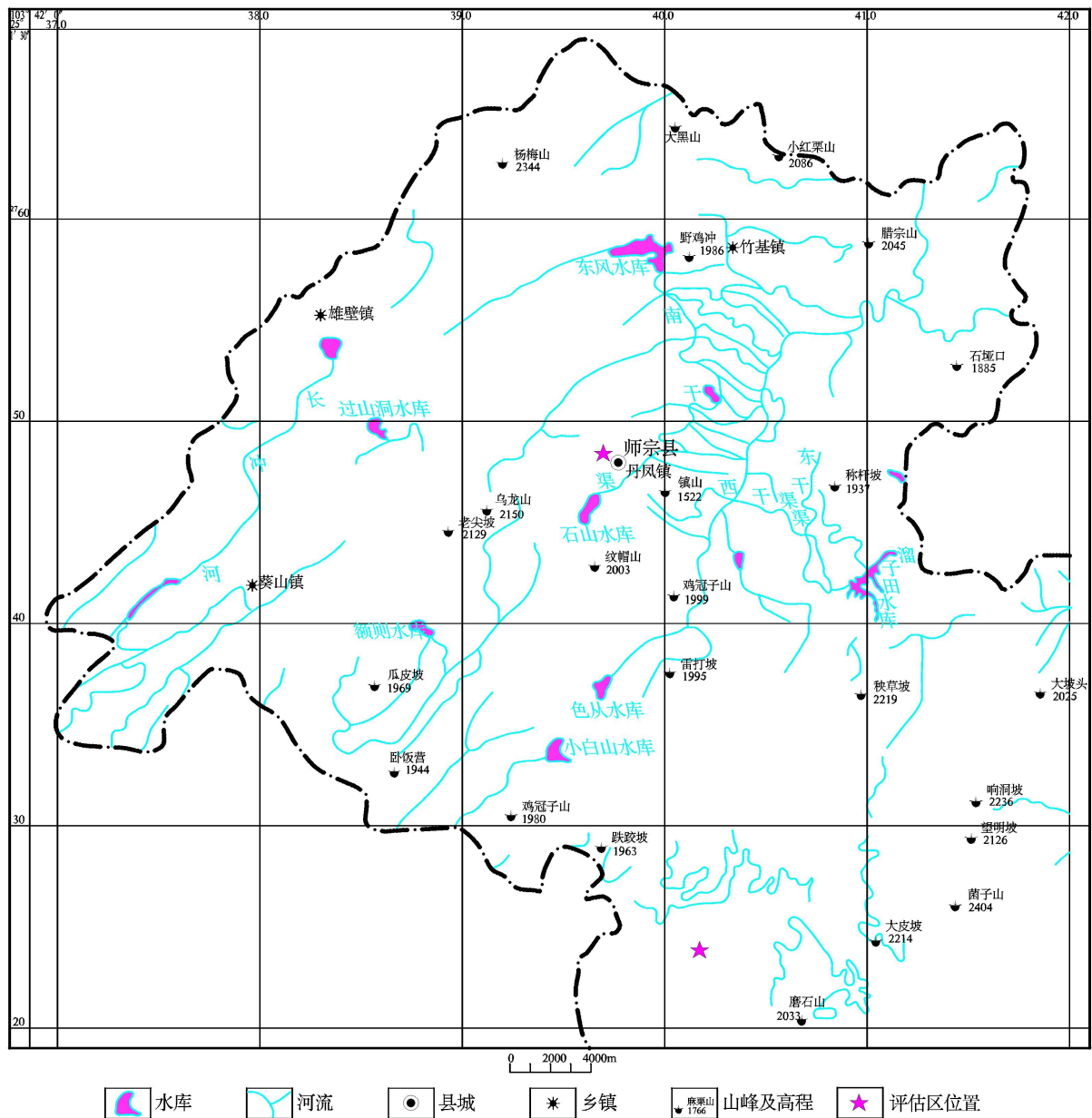
图 2-1 区域水系图
