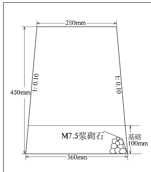
图 5-2 挡土墙断面设计示意图
