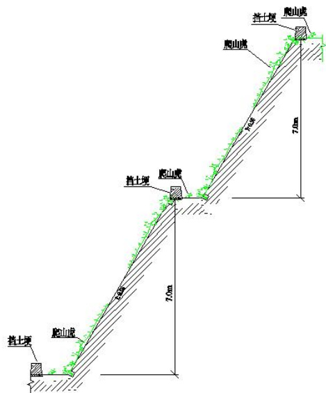
图 5-1 挡土墙示意图
